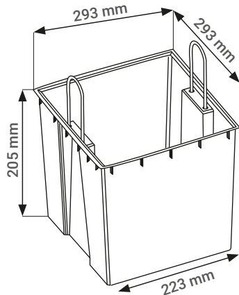
PIC BAC30 Capacidad: 10 l. Recipiente para compartimento de 60 litros, polipropileno 100 % reciclado, asa retráctil. Anillo de acero con recubrimiento en polvo de 1 mm de grosor.
