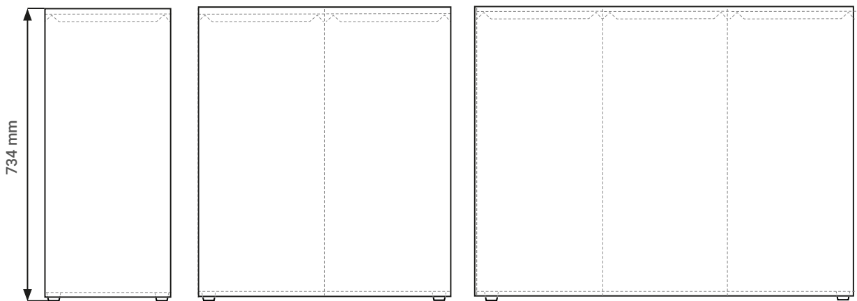
PICW60 SC 1 compartimento 60 L.
