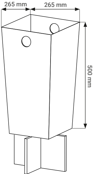
PIC BAC60 Capacidad: 26 litros. Recipiente para compartimento de 60 litros, 100 % polipropileno reciclado. Anillo de PET reciclado.
