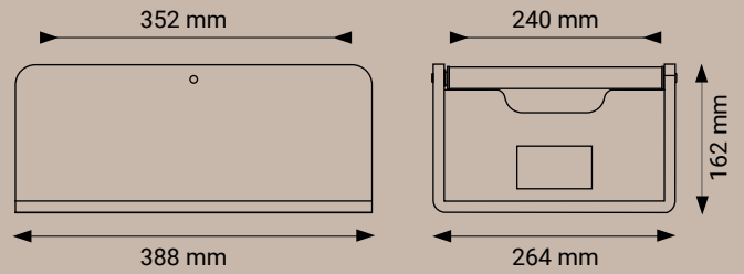
Panier avec 2 poignées orifices Basket with 2 die cut handles
